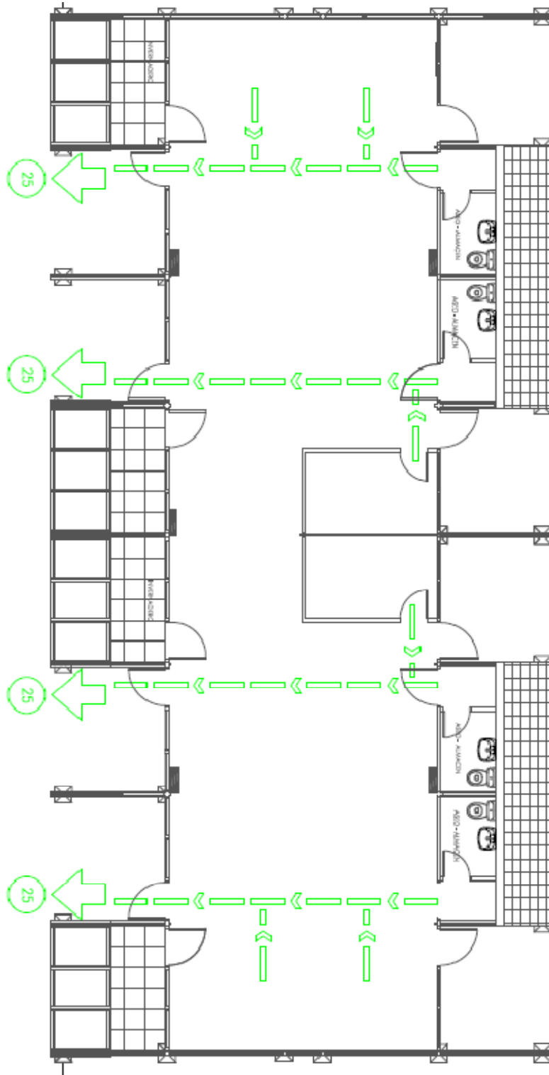
Plano de evacuación de la cabaña Albergue
