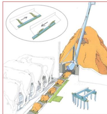
Sistema alternativo con paletas plegables
