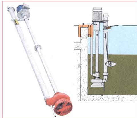
Bomba trituradora vertical
